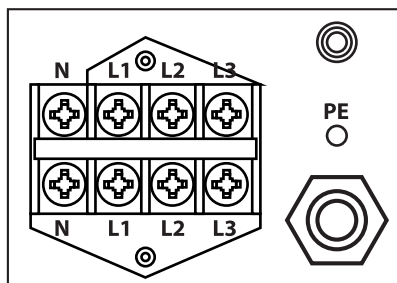
Rysunek 5. Podłączenie urządzenia do instalacji elektrycznej
