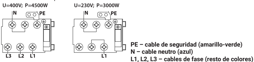
Fig. 2 - Etiqueta de esquema de conexión
