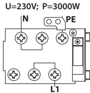
Abb. 2 - Etikette mit dem Schaltplan
