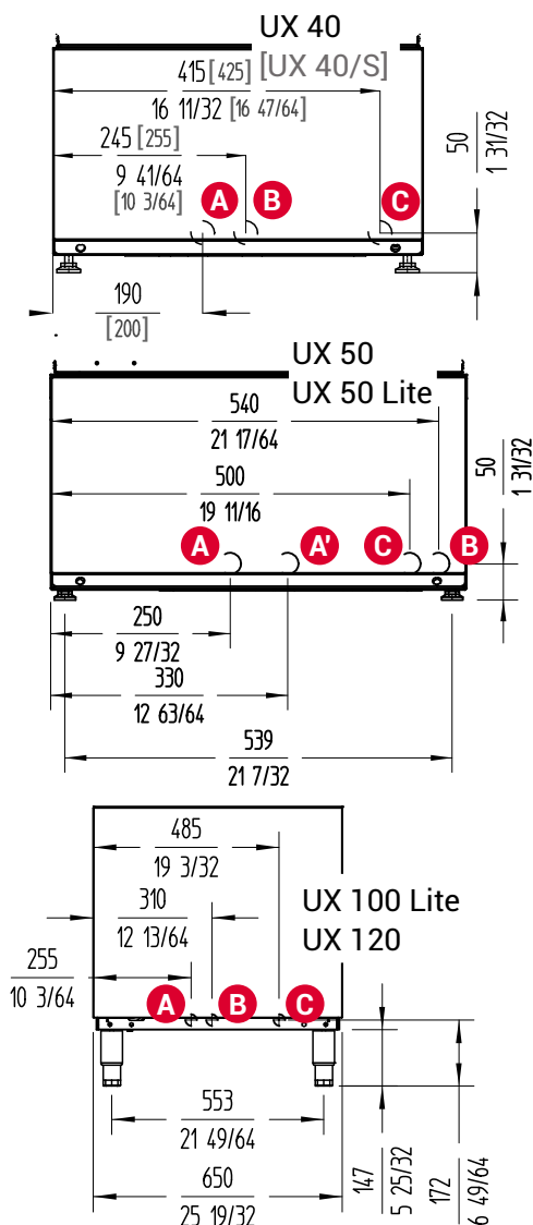
Fig. 1: Pontos de ligação da máquina
