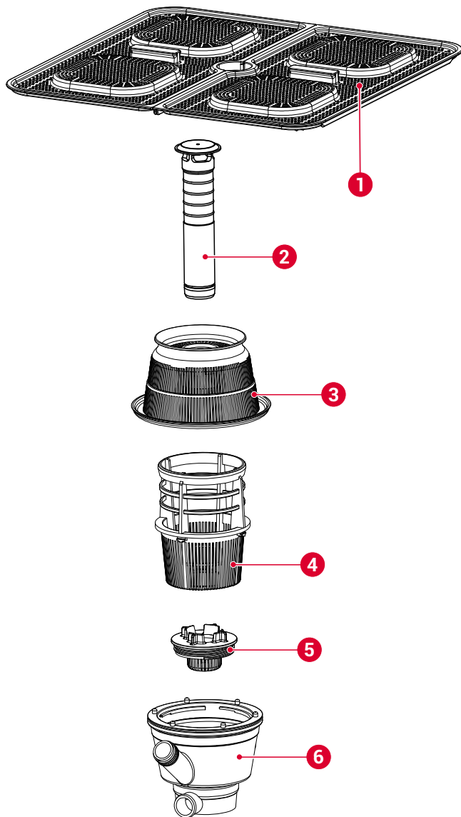
Fig. 4: Filtros da máquina
