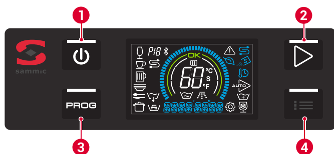
Fig. 2: Pannello di controllo e tasti con LED
