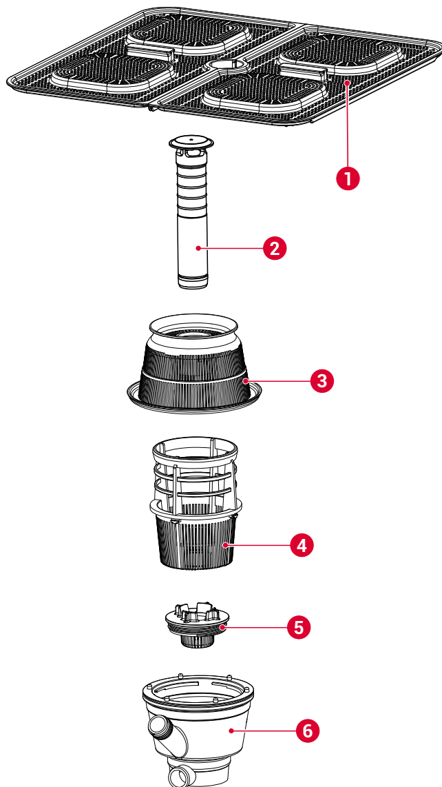
Rys. 4: Filtry urządzenia
