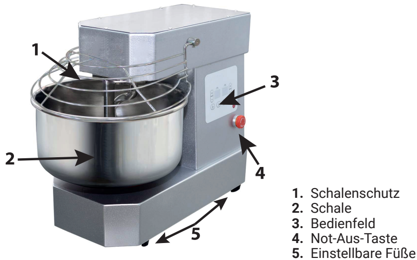
Abbildung 1 Aufbau des Geräts
